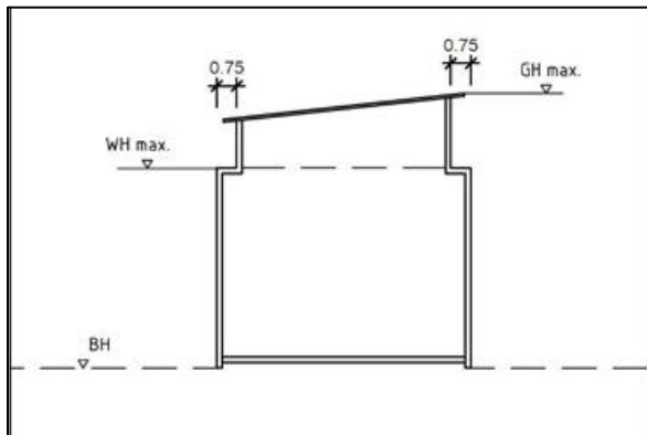
Abbildung 11: Schemaschnitt Staffelgeschoss; Zink Ingenieure
